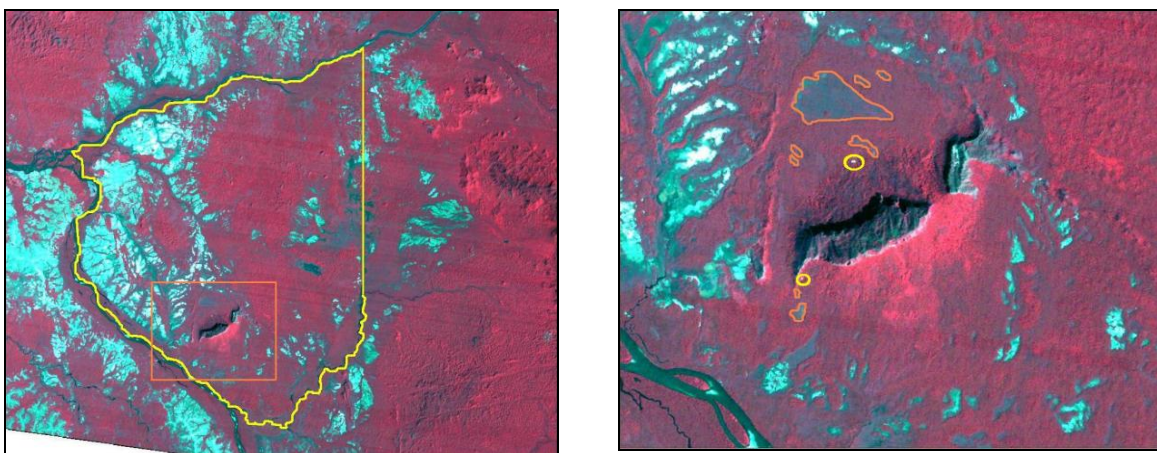
Imágenes Landsat del Parque Nacional Yapacana (izq.) y del Cerro Yapacana (der.) 1991
