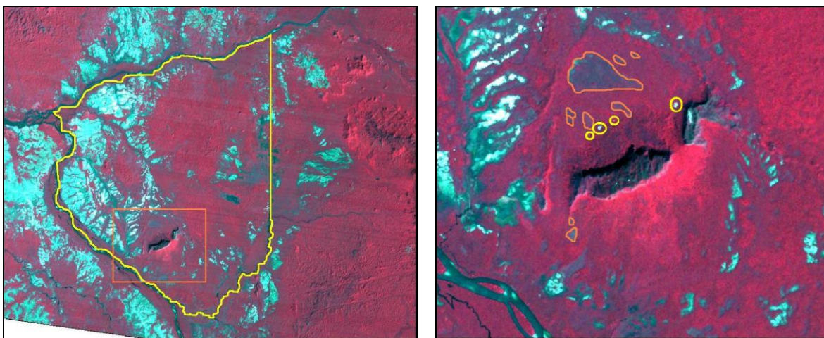
Imágenes Landsat del Parque Nacional Yapacana (izq.) y del Cerro Yapacana (der.) 2000
